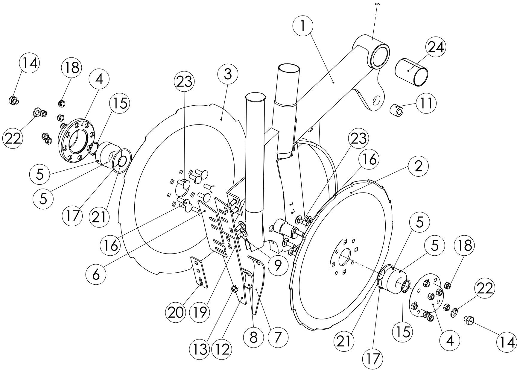
98374802 TAKAVANNAS
