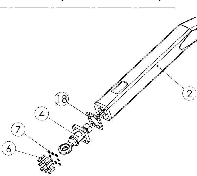
99138403 MUOKKAINVETOAISA
