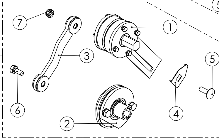
98473004 SÄÄTÖOSAT
