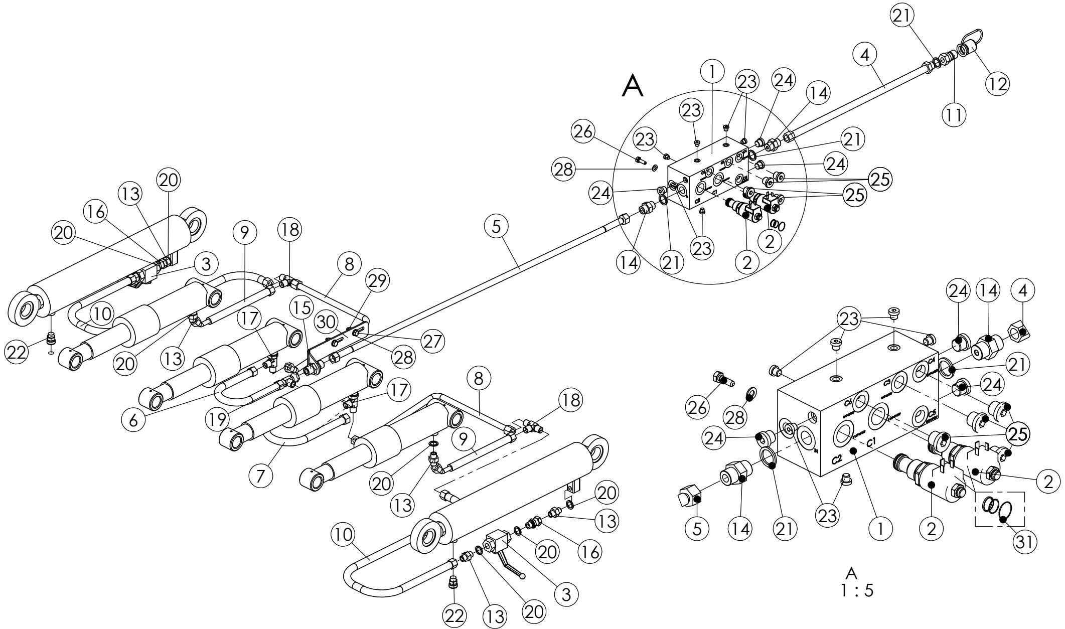
98940602 HYDRAULIIKKA 3000
